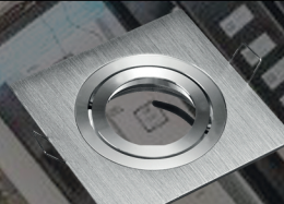
Oprawa sufitowa Jota Średnica wewn.: 80mm Średnica zewn.: 94mm Materiał: Stal Wersja: Srebrna / czarna
