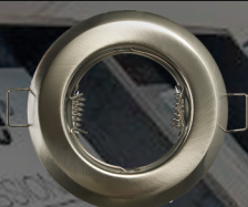
Oprawa sufitowa Alfa Średnica wewn.: 65mm Średnica zewn.: 84mm Materiał: Stal Wersja: Chrom połysk / mat
